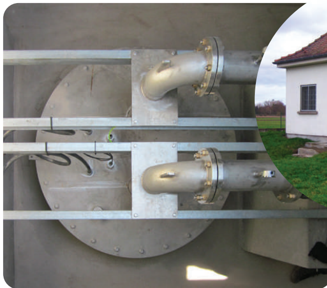
Intérieur et extérieur d'un puit de captage
